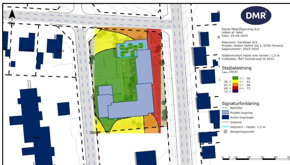
Figur 6.1: Orienterende støjkonturkort for projektområdet, samt punktberegninger på tagterrasse.
