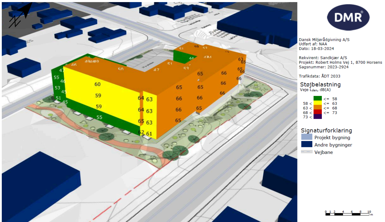
Facadestøjkort - sydøst
